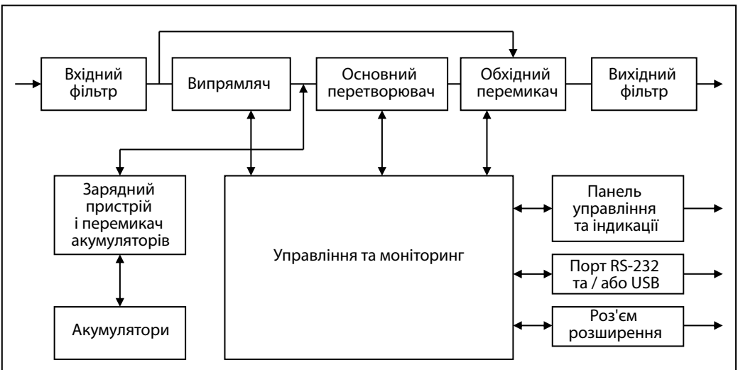
Мал. 7. Блок-схема ДБЖ
