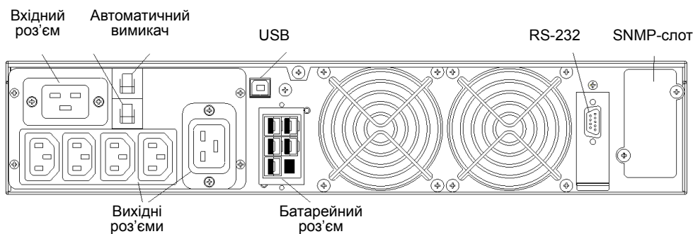
Мал.3. Задня панель серії MRT (1-3 кВА)
